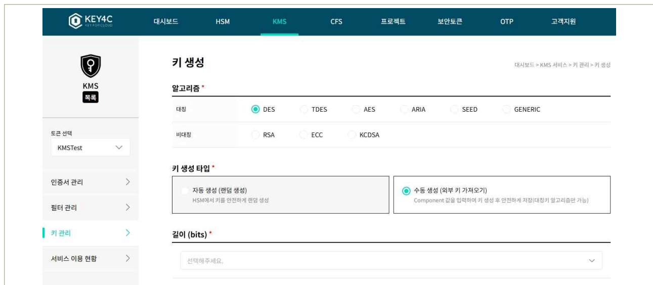
| 그림 4-2-2 | KMS 키 생성 화면
