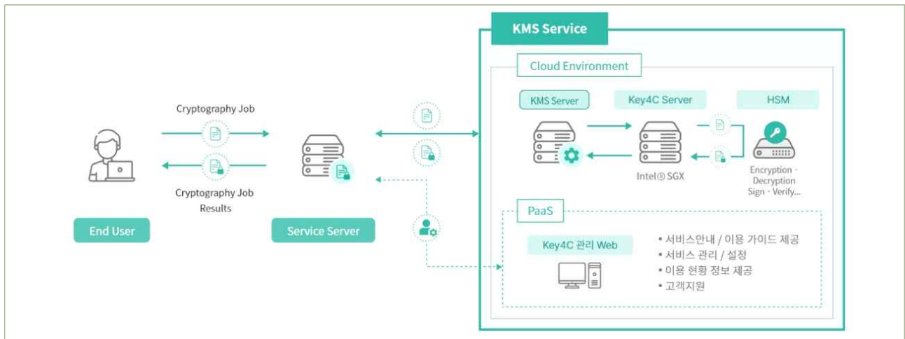
| 그림 4-1-2 | KMS 서비스 개요
