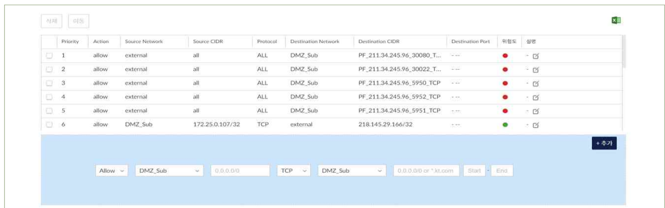
| 그림 2-2-2 | 방화벽 정책 확인, 신규 등록
