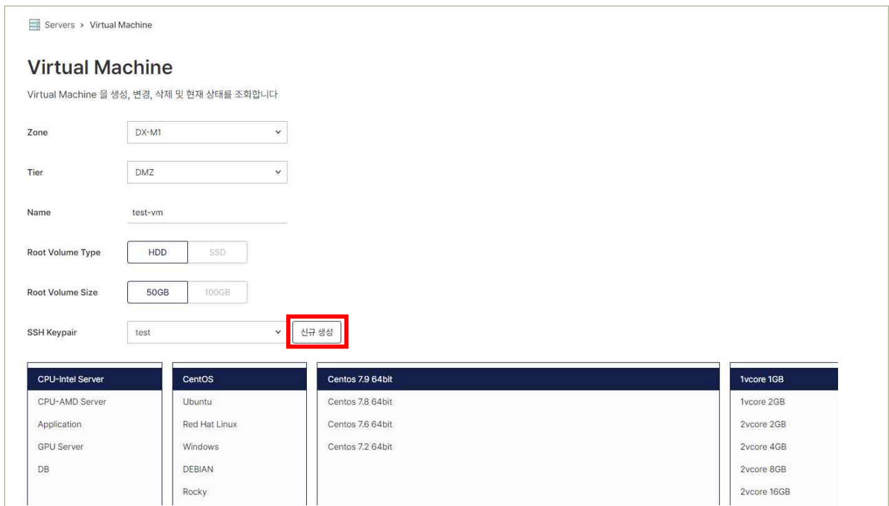
| 그림 1-5-2 | VM 생성 시 SSH Keypair 신규 생성 가능
