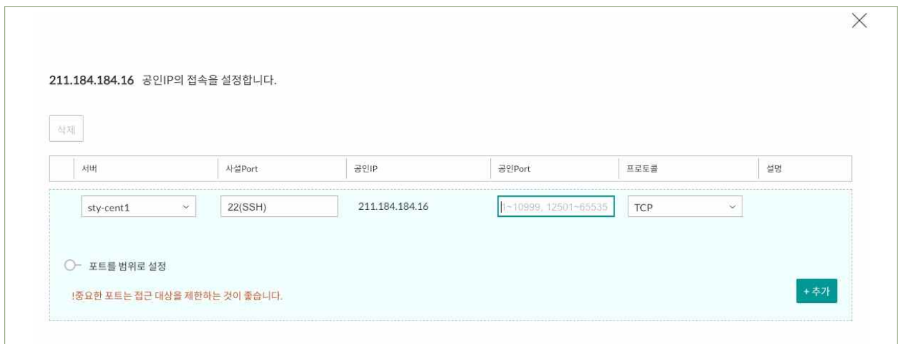
| 그림 1-4-2 | Port-Forwarding 설정 확인
