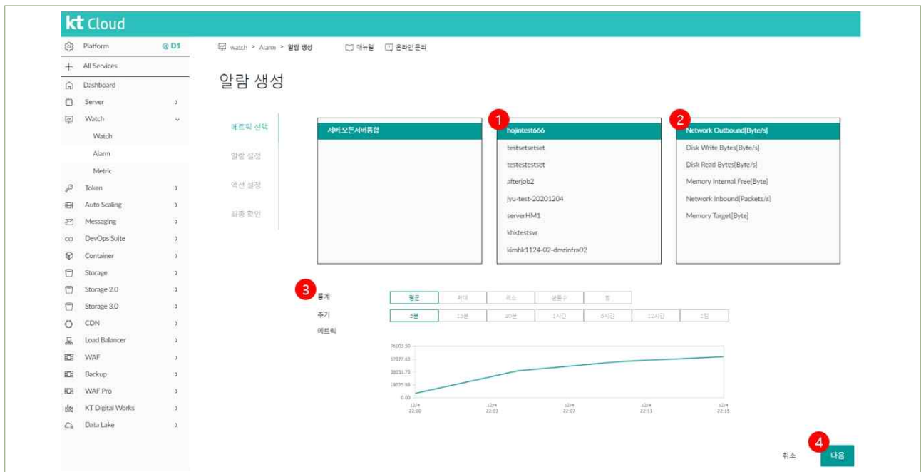
| 그림 5-3-3 | 알람 생성 - 메트릭 선택 화면
