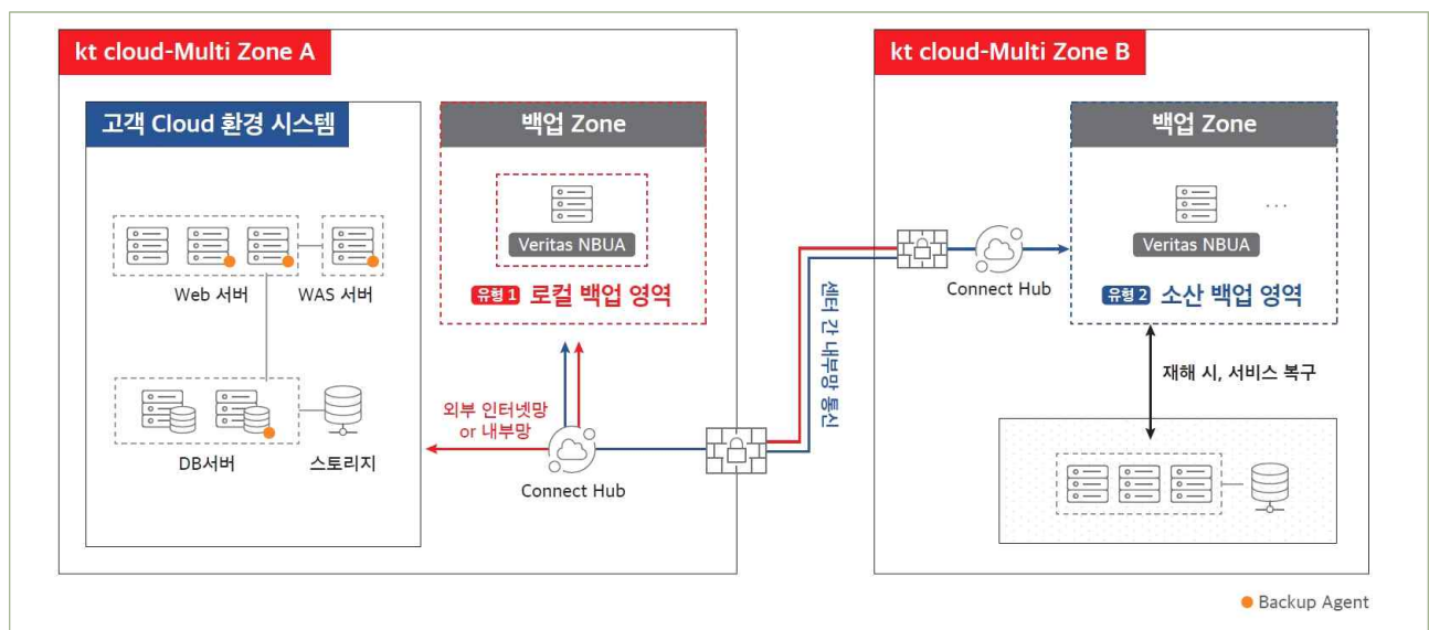
| 그림 8-6-1 | 로컬/소산 백업 구성도
