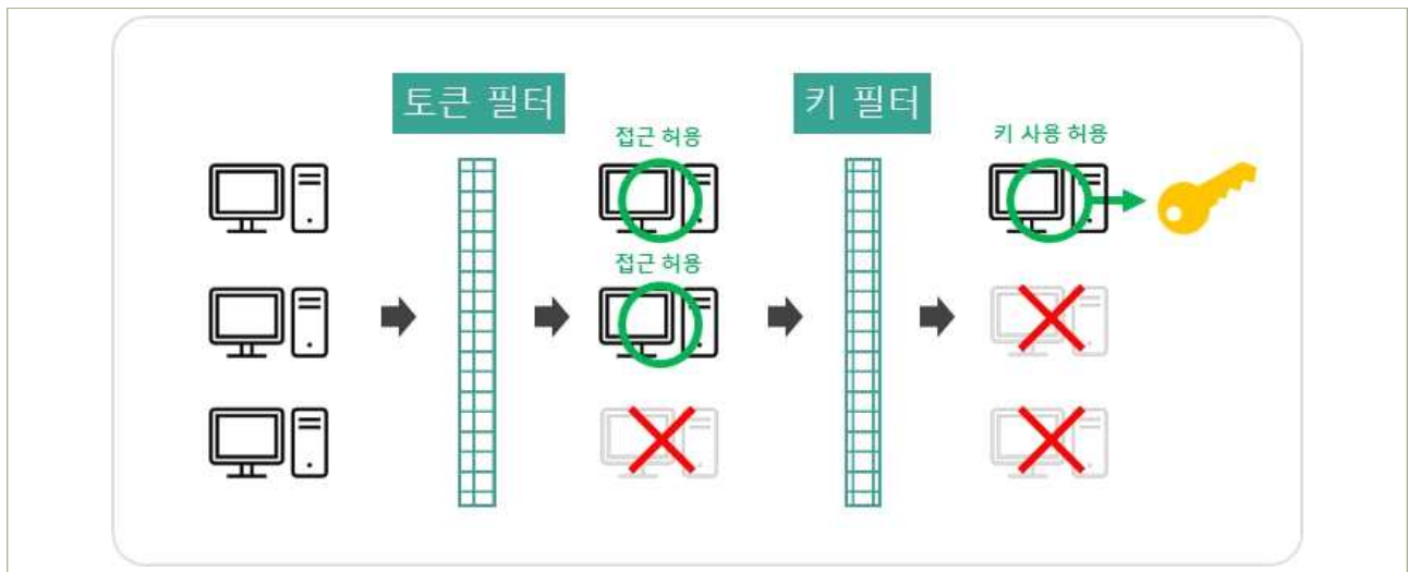
| 그림 4-4-1 | KMS 필터(접근제한) 개념
