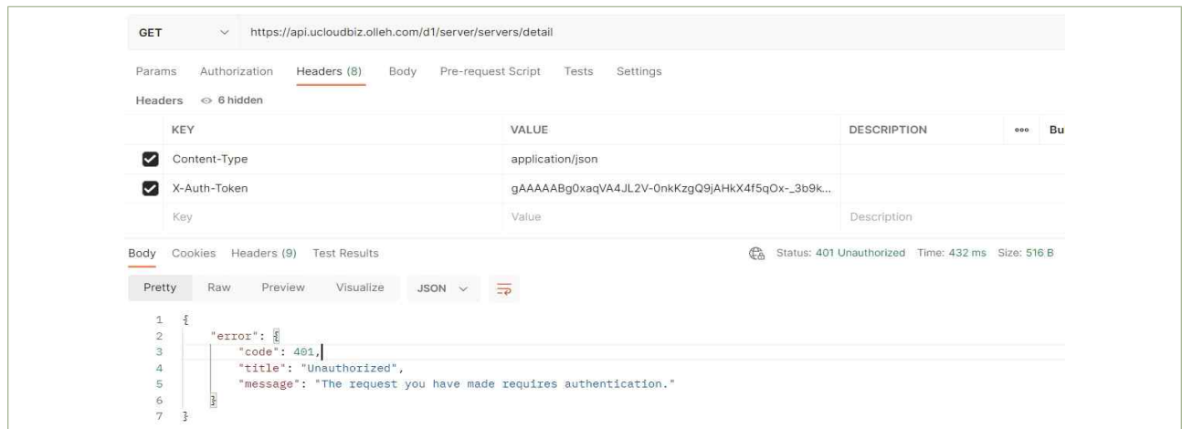
| 그림 6-4-1 | 만료된 토큰으로 API 실행
