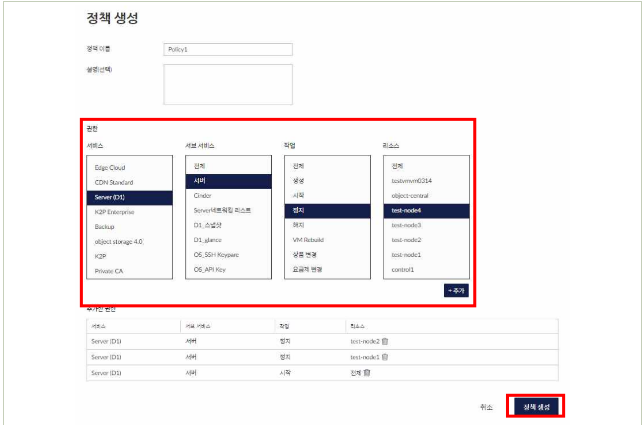
| 그림 3-1-2 | 사용자 권한 관리를 위한 정책 생성
