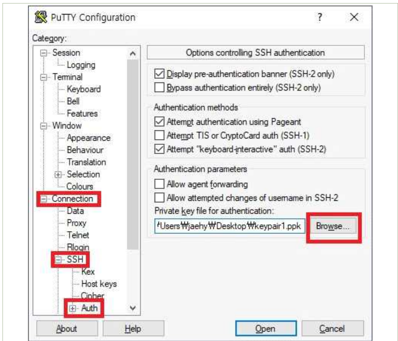
| 그림 1-1-6 | SSH 접속 시 Keypair를 이용 방법
