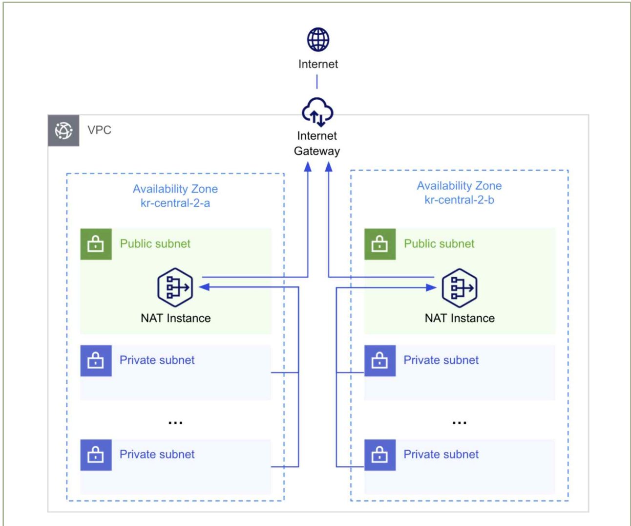
| 그림 2-2-15 | NAT 인스턴스 구성 예시 아키텍처
